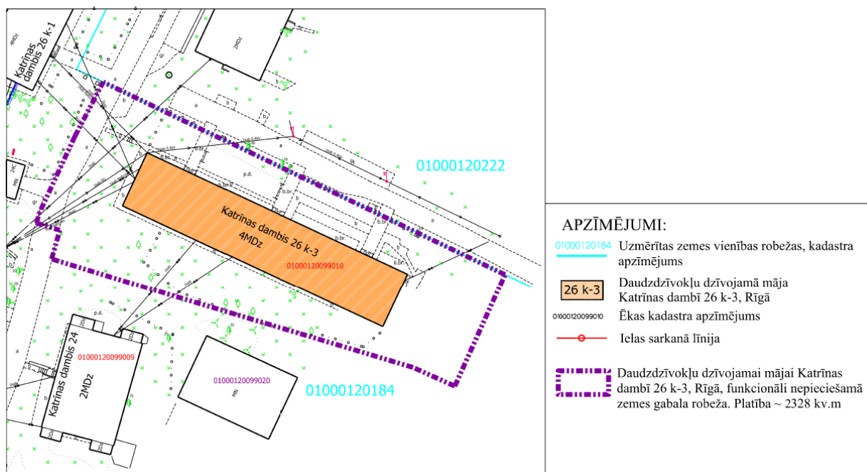
2.attēls Daudzdzīvokļu dzīvojamai mājai Katrīnas dambī 26k-3, Rīgā, funkcionāli nepieciešamā zemesgabala robeža
